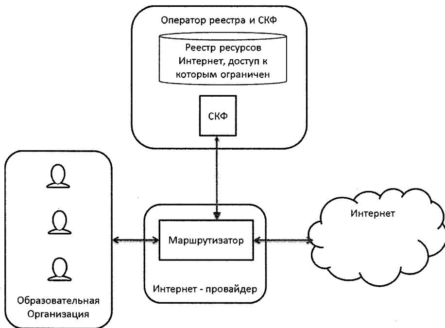
Рисунок 5. Схема работы контент-фильтрации при едином решении
