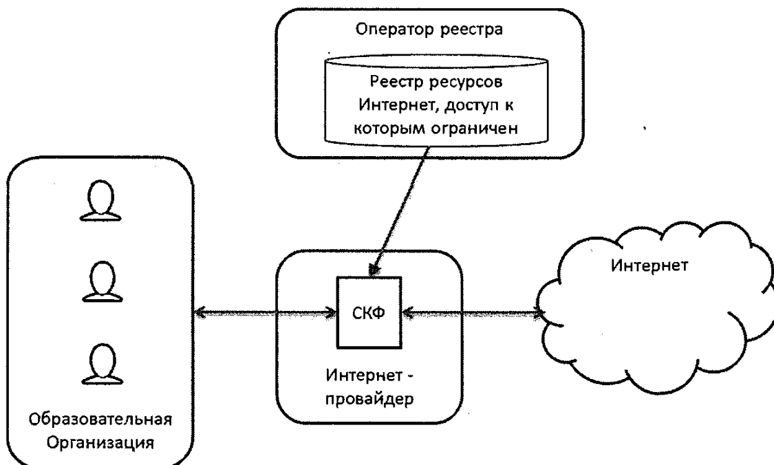
Рисунок 4. Схема работы контент-фильтрации при размещении у Интернет-провайдера
